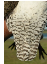
Archibebe común
